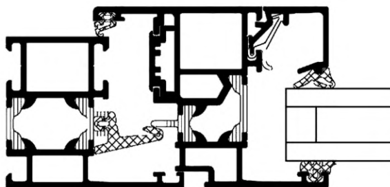
б) Комбинированные профили с однокамерной термоизоляционной вставкой
