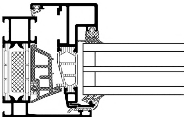
в) Комбинированные профили с многокамерной термоизоляционной вставкой
