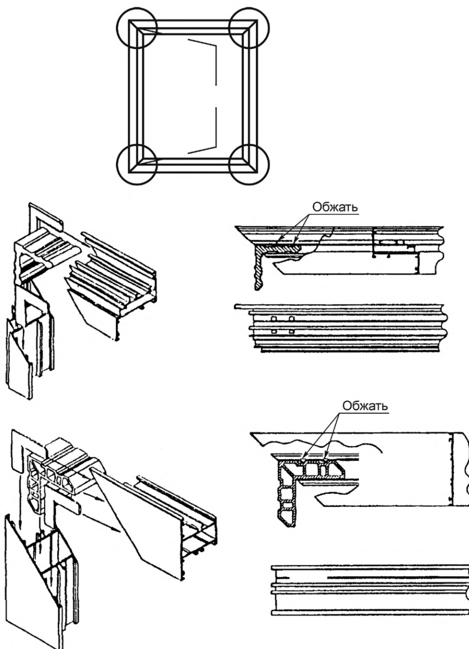
Рисунок А.2 — Примеры конструкции узлов угловых соединений створки и коробки
