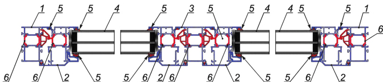
Рисунок 5 — Пример конструктивного решения алюминиевого двухстворчатого оконного блока с импостным притвором
