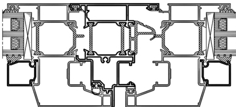
Рисунок 6 — Пример конструктивного решения штапикового притвора
