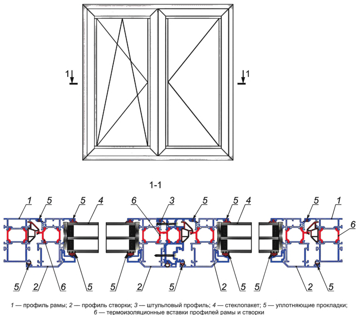
Рисунок 7— Пример конструктивного решения алюминиевого двухстворчатого оконного блока со штапиковым притвором
